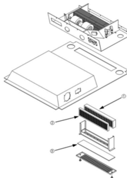
Filtros de aire fresco de la cabina • (1) – Filtro de papel • (2) – Filtro de carbón • (3) – Filtro de recirculación -Vista típica
