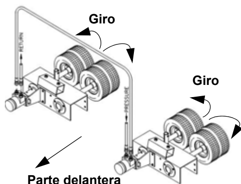
Parte delantera Conjunto hidráulico de extractores cuádruples (modelo de dos cabezales) -Vista típica
