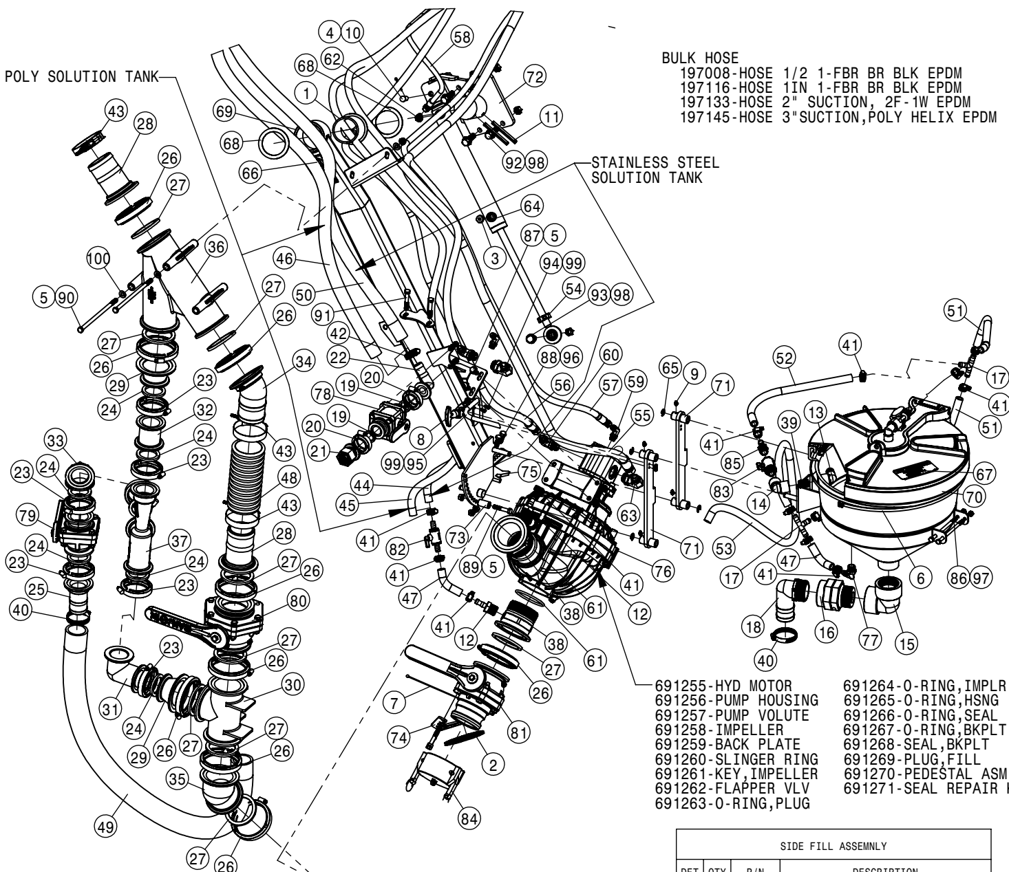
SIDE FILL ASSEMBLY
