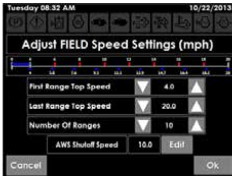
Mezei sebességek beszabályozásának képernyője
