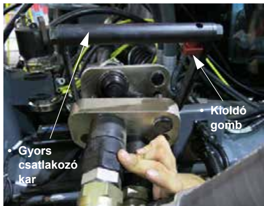
Hidraulikus multi-csatlakozó összeszerelés (a gép jobb oldalánál helyezkedik el) – Tipikus nézet
