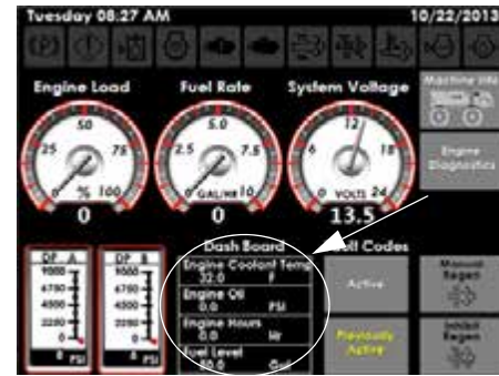
Rendszerdiagnostika (a gépdiaosztikái oldalon)
