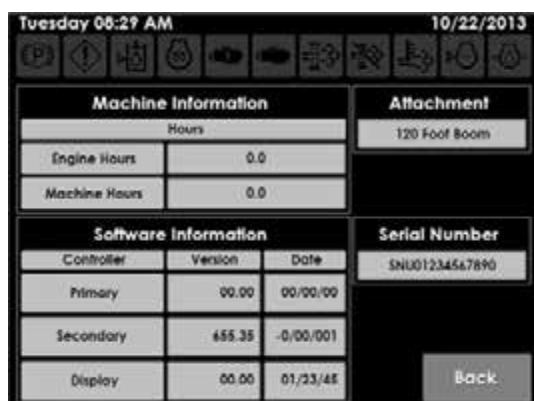
Ecran Informații utilaj
