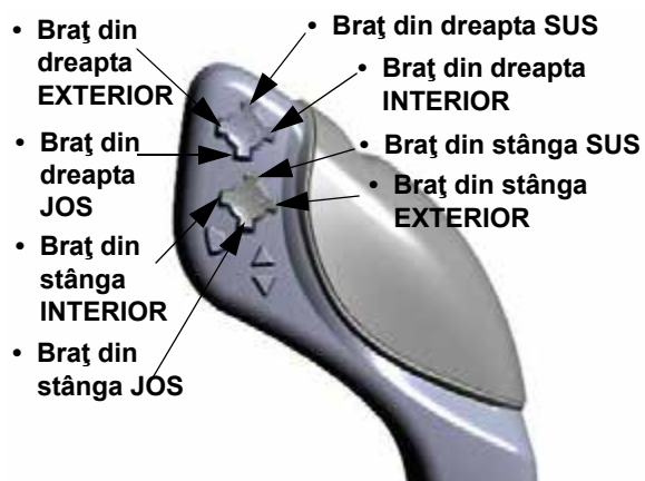
Orientare comutator brațe din stânga și din dreapta - Vedere tipică
