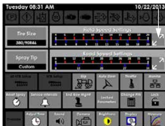
Buton de reglare pentru setările de viteză în modul Câmp (amplasat pe pagina Setări)
