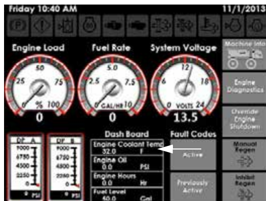
Indicatorul de temperatură pentru agentul de răcire a motorului (amplasat pe pagina Diagnoză utilaj)
