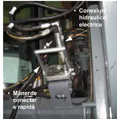
• Conexiuni hidraulice/electrice • Mâner de conectare rapidă Ansamblu cuplaj multiplu hidraulic/electric - „dacă este prevăzut cu această componentă” (amplasat pe partea din stânga față a utilajului)
