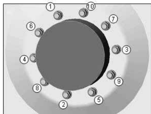
Очередность затяжки
