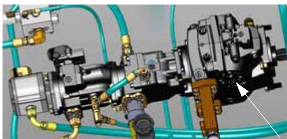
Hidrosztatikus szivattyú (hajtás szivattyú) – Tipikus néze (A berendezés felülnézete)
